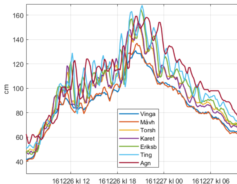
Figur 4. Vattenståndet under stormen Urd. Här visas vattenståndskurvorna för alla mätlokaler. Seichen syns tydligt på mätlokalerna i Älven: Eriksberg, Tingstad och Agnesberg. Karet och Torshamnen ligger strax utanför älvmynnningen. Seichen syns tydligt även där, men har lägre amplitud. Den är knappt synlig vid Måvholmsbådan fem km ut. Vid Vinga, 12 km ut, är seicheamplituden försvinnande liten.
